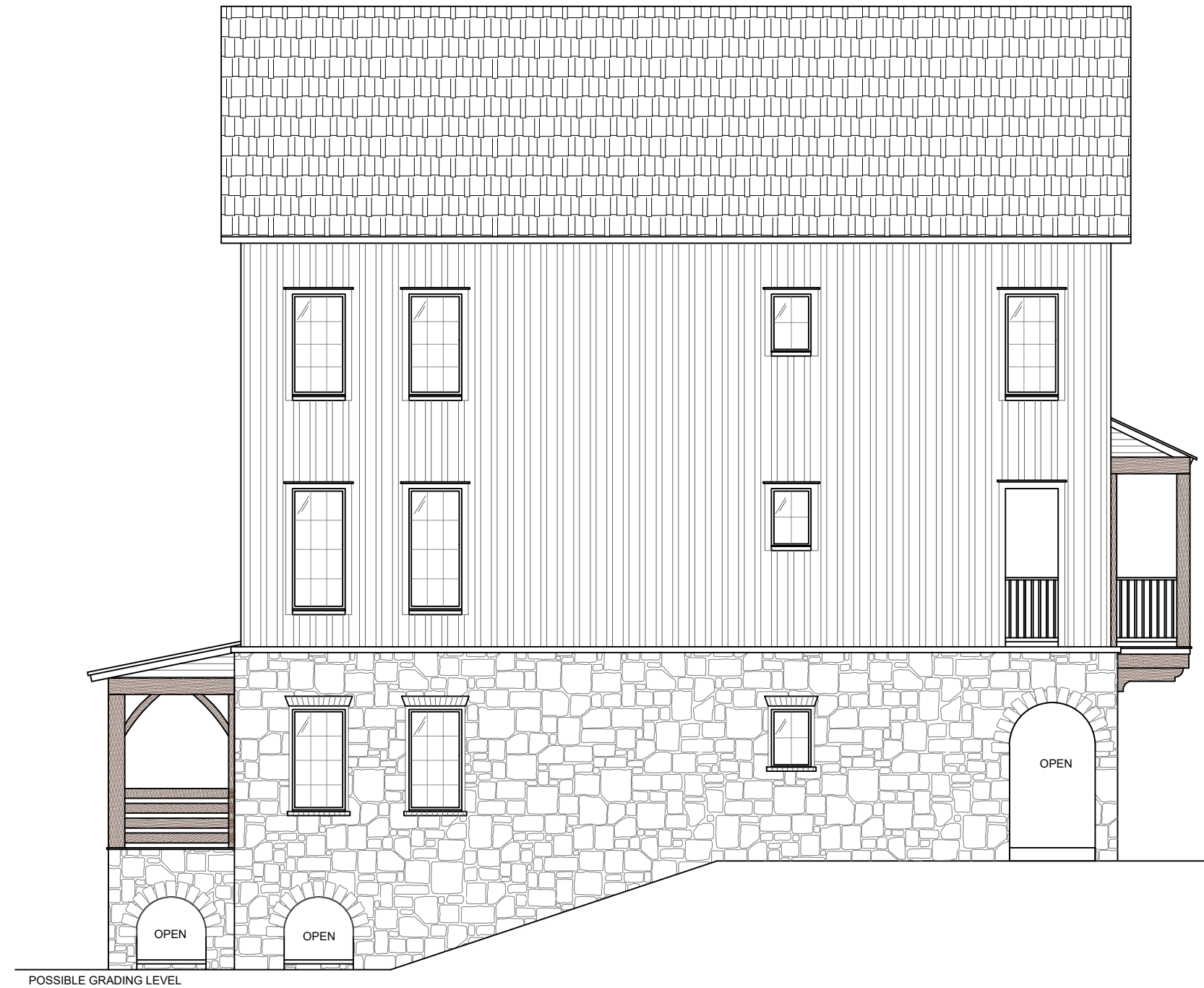
Right Elevation
